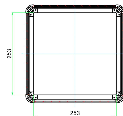
C-C ( 1 : 5.5 )
