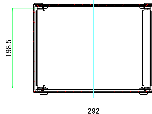
B-B ( 1 : 5.5 )
